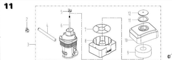
Silnik spalinowy HGS ST 255 HS 208 (170 F)
